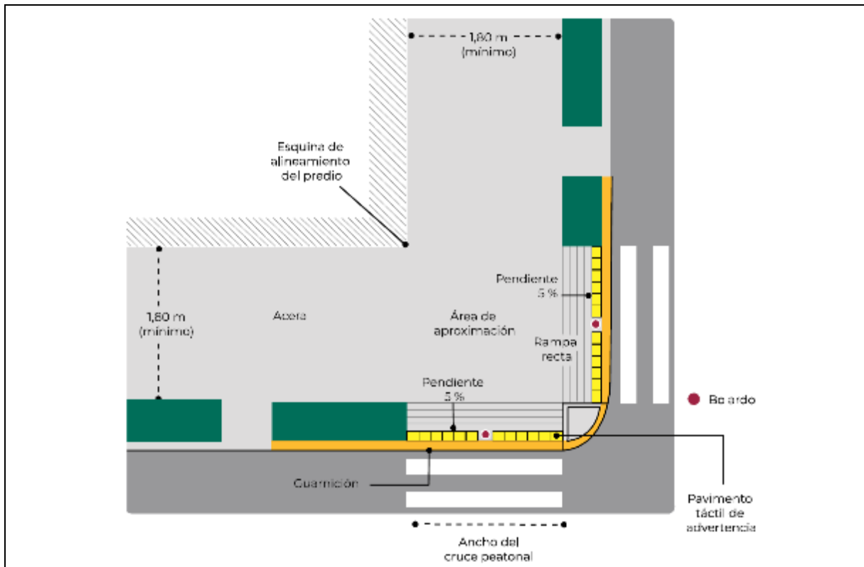
Figura 35.- Rampas rectas, variante 1 (planta) [1] [2]
