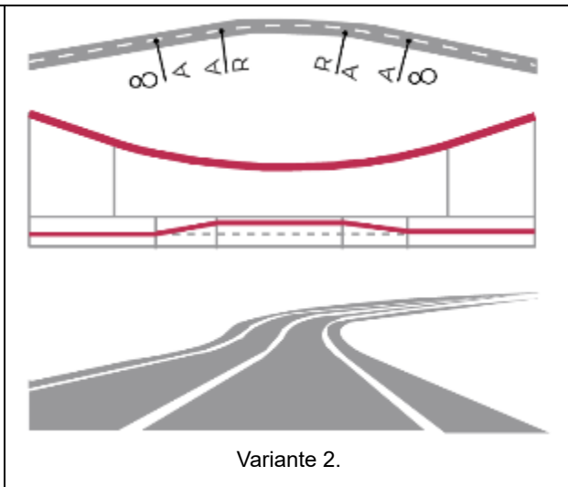
Figura 20.- Acentuada desproporción entre elementos de trazo [1] [2]
