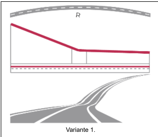
Figura 20.- Acentuada desproporción entre elementos de trazo [1] [2]
