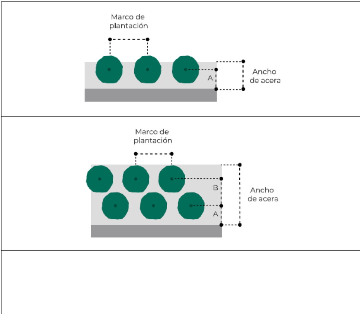
Figura 110.- Dimensiones de referencia para la colocación de árboles en las banquetas. [1] [2]
